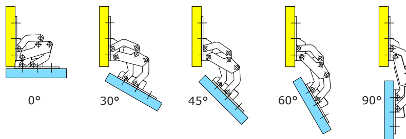
Exemple de montage porte en applique
