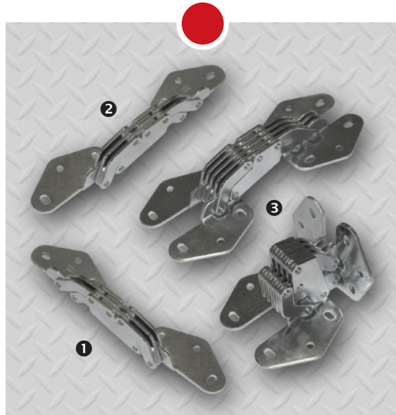
Charnière ❶ 70-1-3527 (O), ❷ 70-1-3528 (O), ❸ 70-1-3303 (Ouvert et Fermé)
